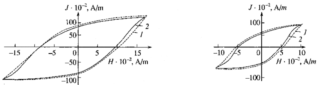
Рис.1. Экспериментальные (1) и расчетные (2) кривые намагничивания для двух марок стали: АК-29 и АК-32 (левый и правый графики соответственно).
