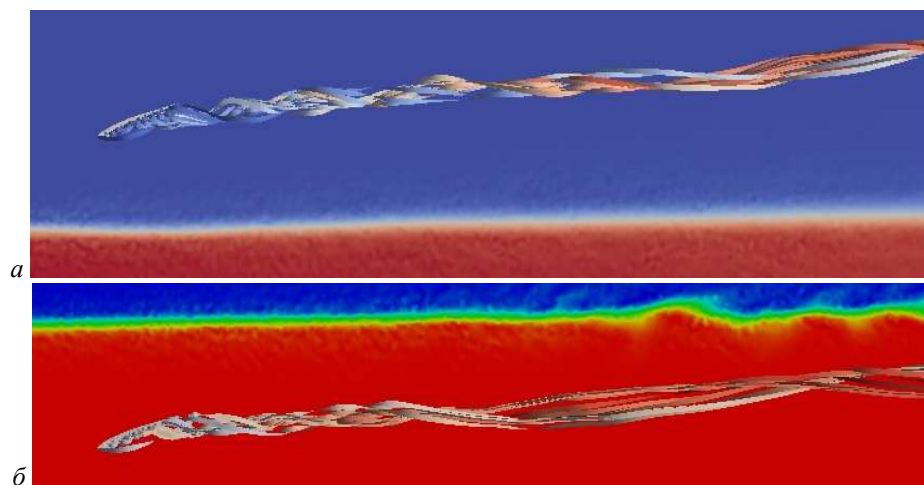
Рис.2. Взаимодействие вихревого следа крыла с пикноклином.
