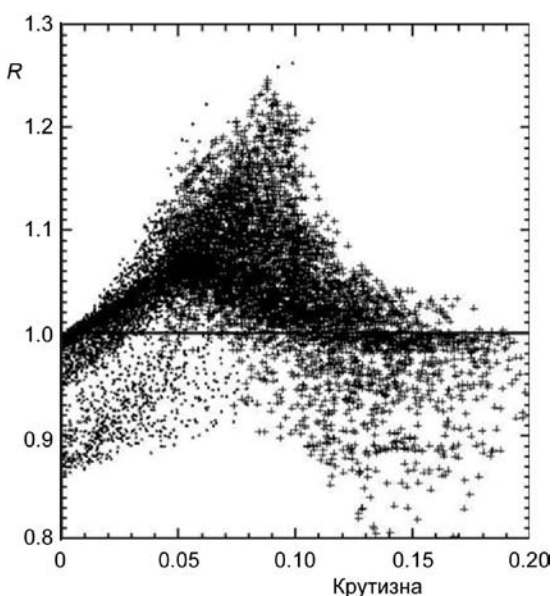
Рис. 5. Зависимость параметра превышения от крутизны заданного в начальных условиях волнового поля. Случаи опрокидывания отмечены знаком +; случаи, когда опрокидывание не произошло за первые 10 периодов — точкой.
