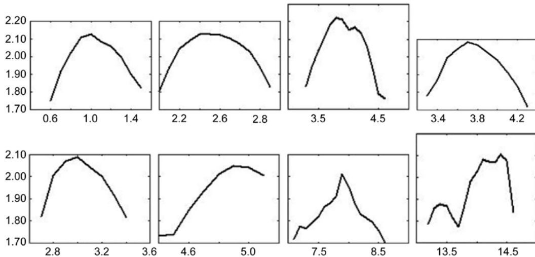
Рис. 3. Лагранжева эволюция высоты экстремальных волн (нормированная высотой значительной волны), рассчитанная в численных экспериментах с трехмерной моделью. Горизонтальная ось соответствует времени, выраженном в периодах волны пика.
