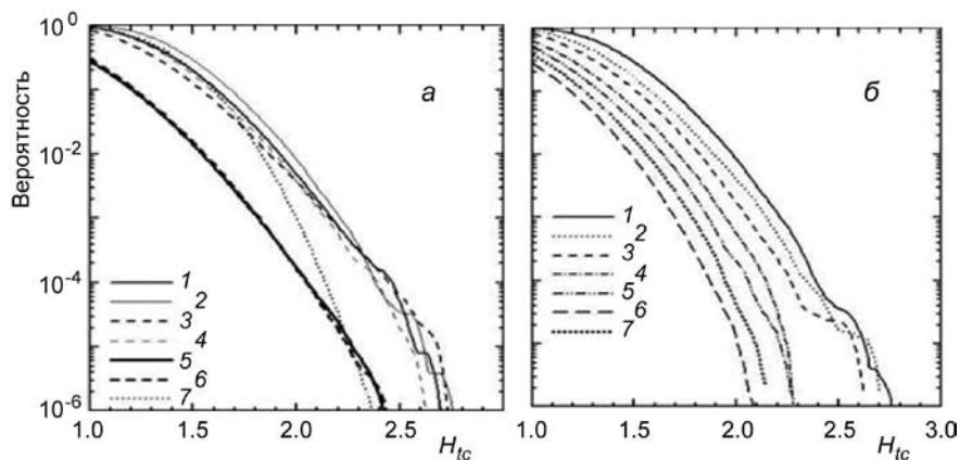
Рис. 4. Повторяемость высоты волны от подошвы до гребня.
